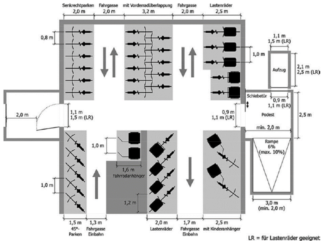
Grafik 2: Mindestmaße für eine ebenerdige Fahrradaufstellung und Zufahrten bzw. Zugänge; Vgl.: RVS 03.02.13, S. 81
